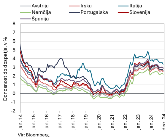
Slika 26: Obveznice, 4. četrletje 2024
