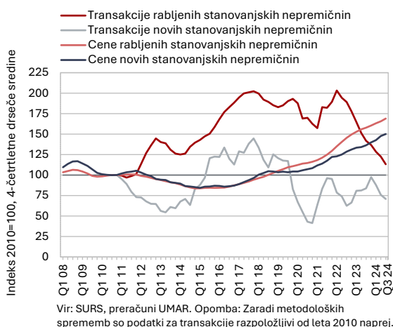
Slika 16: Nepremičnine, 3. četrletje 2024
